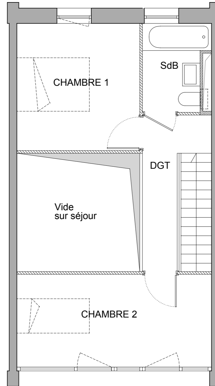
L3 - Version 1 - Haut Duplex
